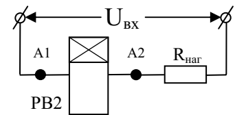
Рис.3 Схема включения реле на активную нагрузку
