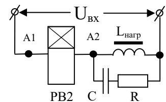
Рис. 4 Схема включения реле на индуктивную нагрузку (катушку пускателя и т.п.), где:
