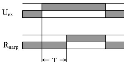
Рис.5 Временная диаграмма работы реле времени
