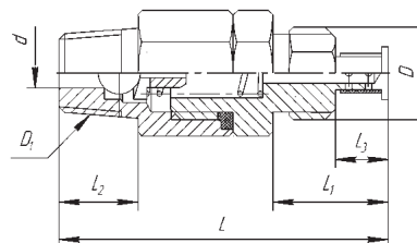
Клапан обратный НKK-4
