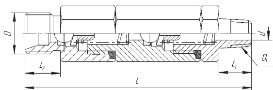
Клапан обратный НKK-5
