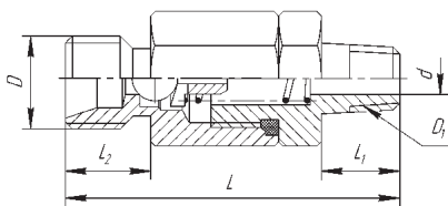
Клапан обратный НKK-2
