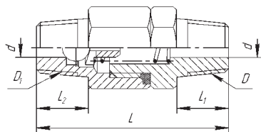
Клапан обратный НKK-1
