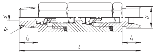
Клапан обратный НKK-3
