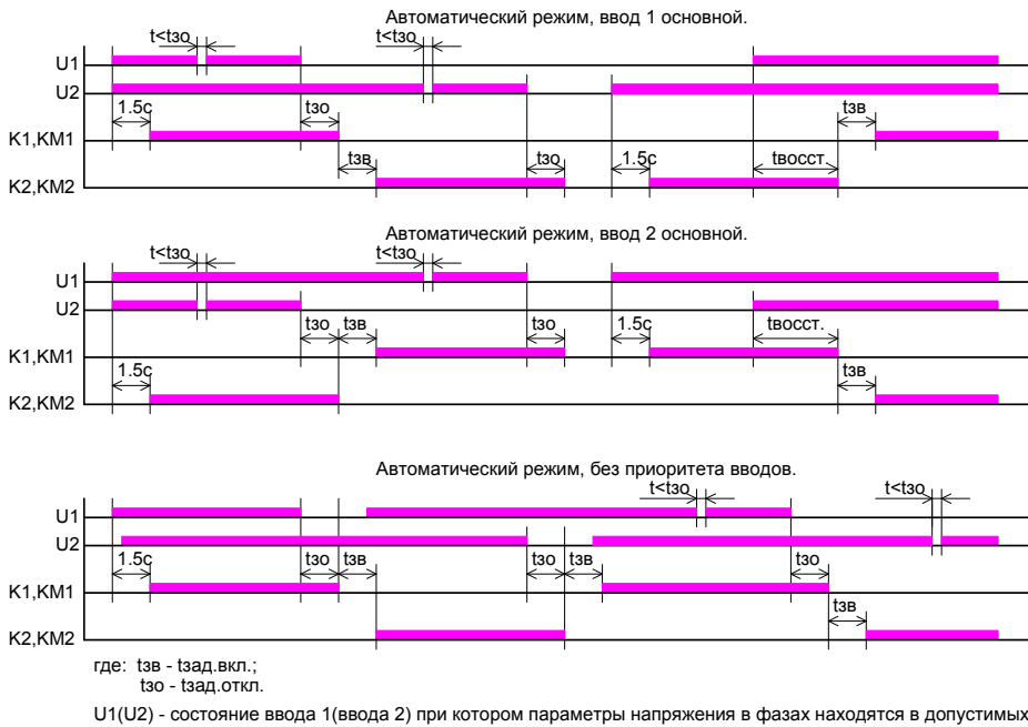
Рис.3 Схема и временные диаграммы работы АВР на магнитных пускателях с двумя вводами, одной группой нагрузок, с электрической блокировкой магнитных пускателей и управлением от БУАВР1.х.х
