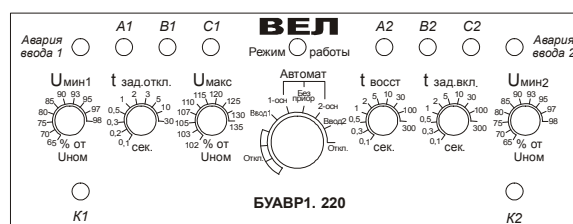
Рис. 2 Расположение органов управления и индикации БУАВР1
